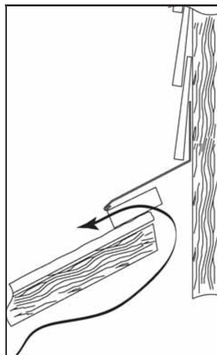
Вентиляция на примыкании
